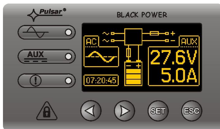
Rys. 5. Panel kontrolny.
