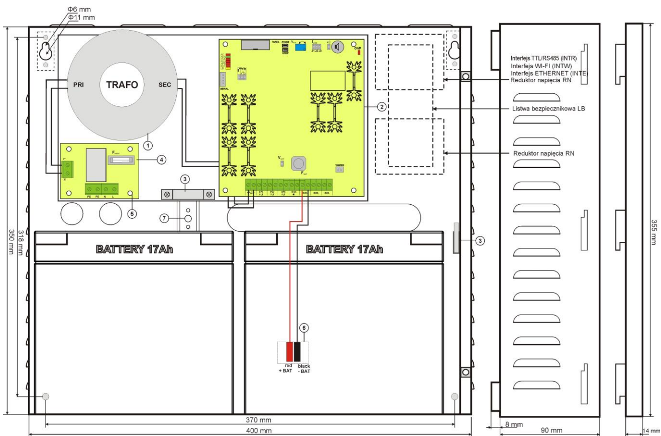
Rys.3. Widok zasilacza.
